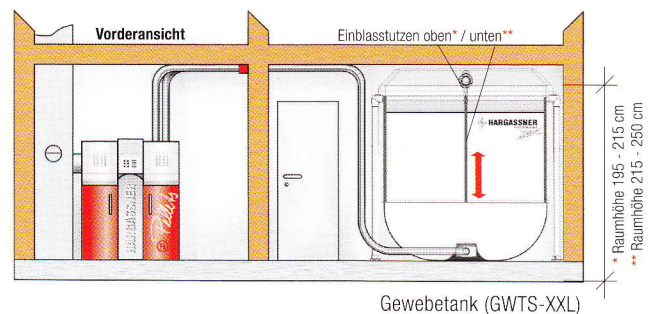
Gewebetank (GWTS-XXL)
